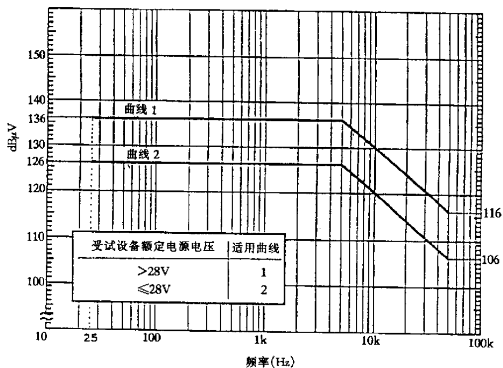
图 CS101-1 CS101 极限(AC 和 DC)
