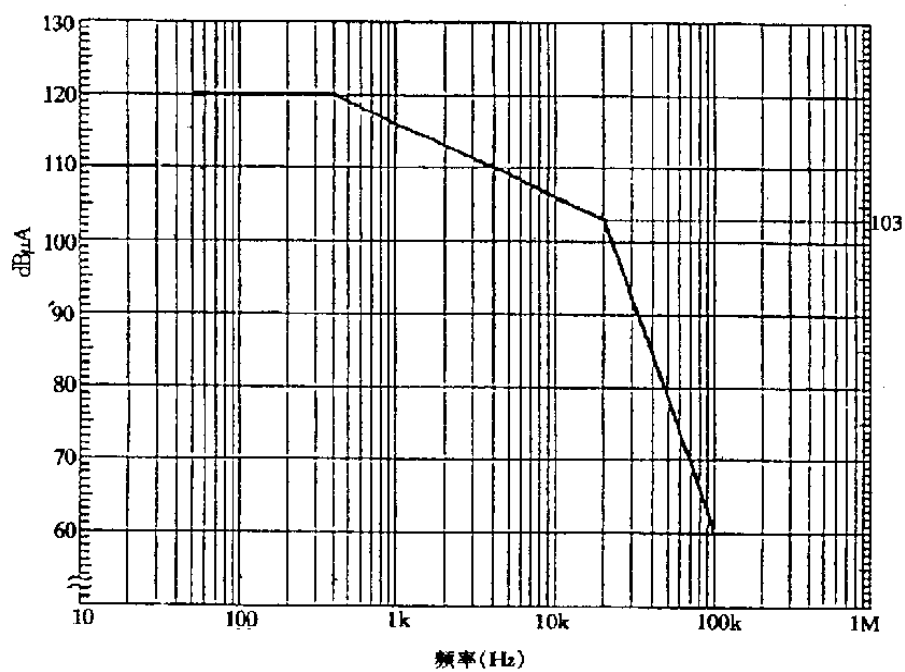
图 CS109-1 CS109 极限
