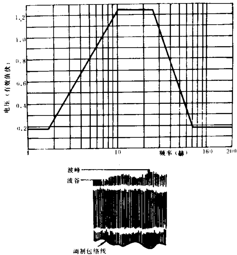
图4 电压调制频率特性极限
