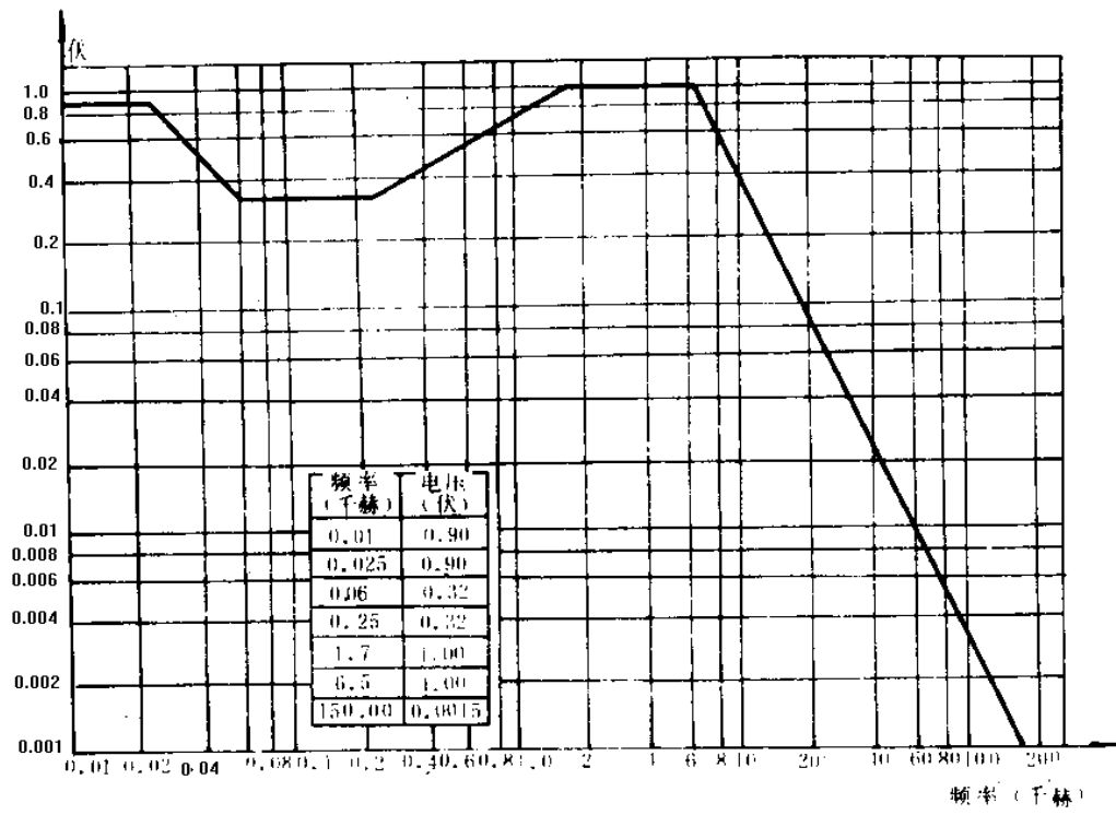
图9 直流供电系统脉动电压频谱范围
