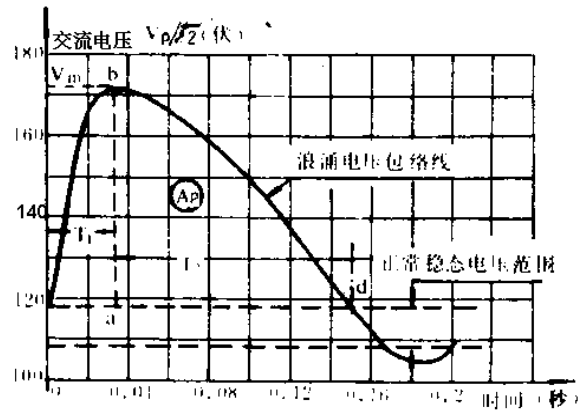
图 17 过压浪涌转换成等值阶跃电压
