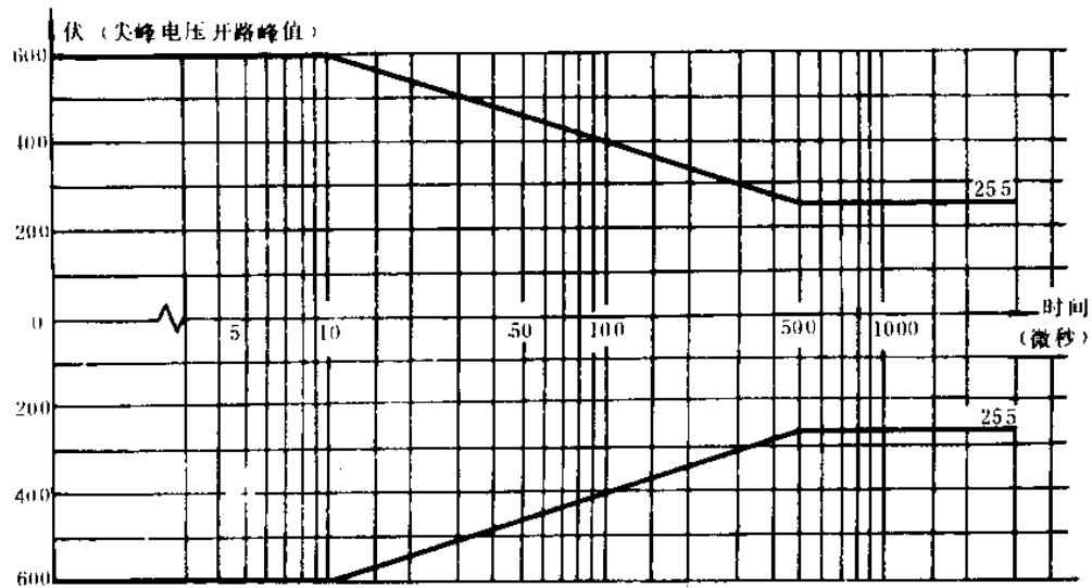
图3 交流用电设备产生尖峰电压极限
