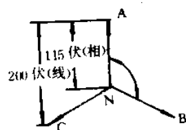
图 1 相序图
