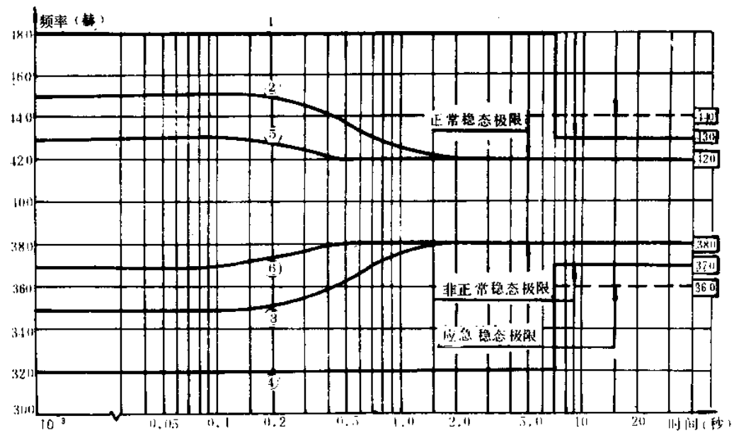
图8 瞬态频率极限曲线
