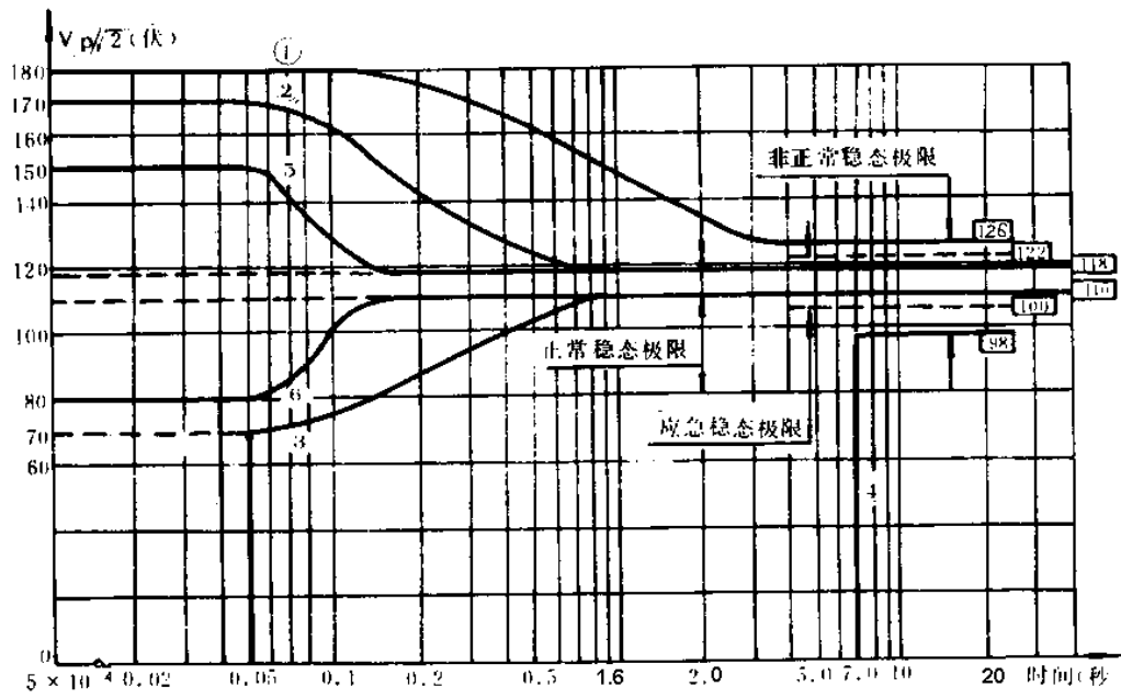
图5 交流A类供电浪涌等值阶跃电压极限曲线
